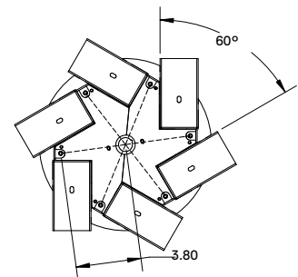
F6 - 6 Fixture Fan
